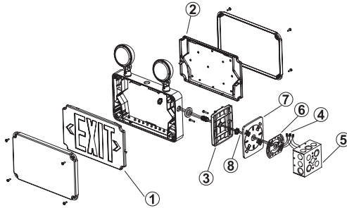
Mini Wet Location Exit Combo
