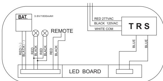
COMBO RC Wiring Diagram:
