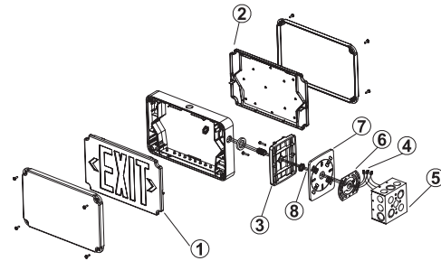
Mini Wet Location Exit Sing
