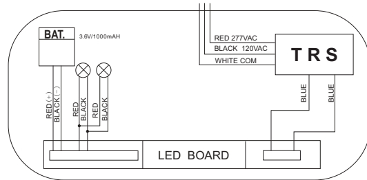
COMBO Wiring Diagram:
